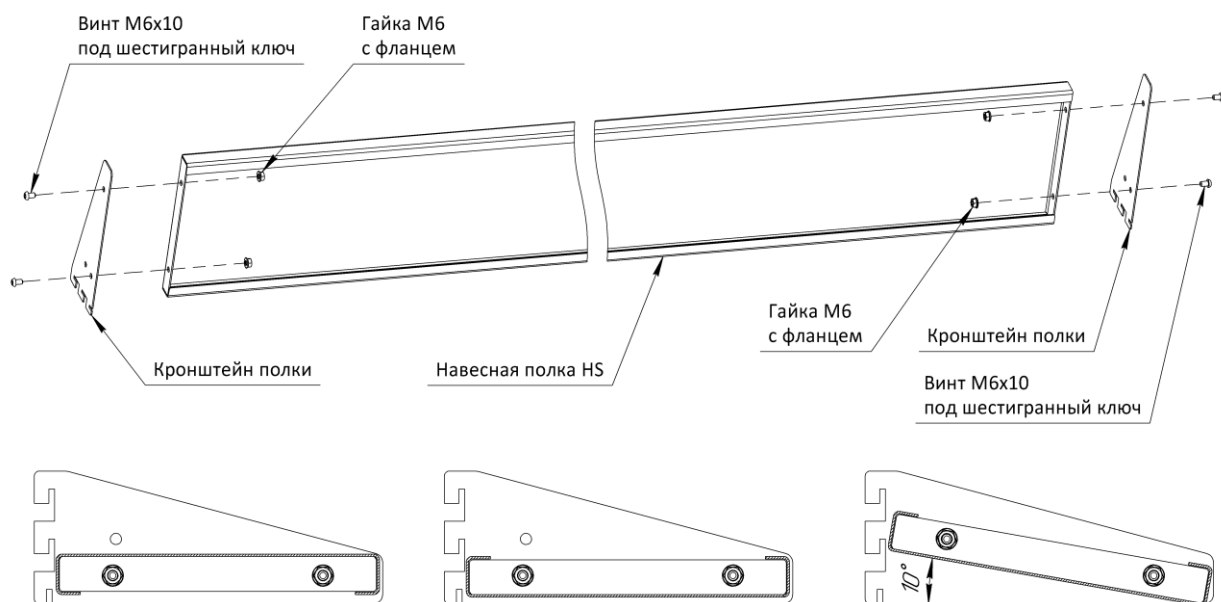
Варианты установки навесной полки
