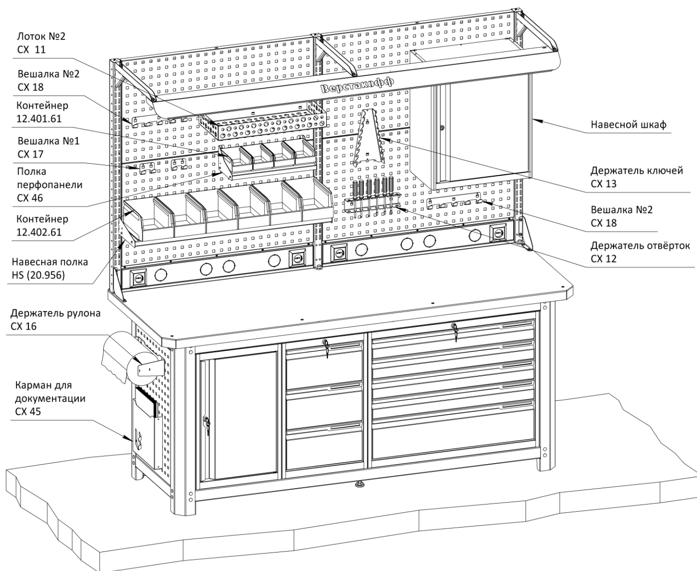
Пример наполнения верстака MCN 2052.S73L5-2FR аксессуарами
