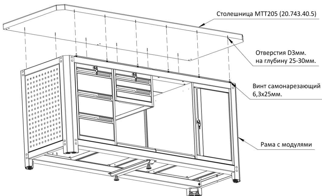
Крепление столешницы к раме
